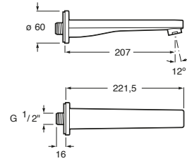
Escuadra Wall Bath Outlet
