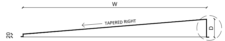
TEGO® MODULE SIZES
