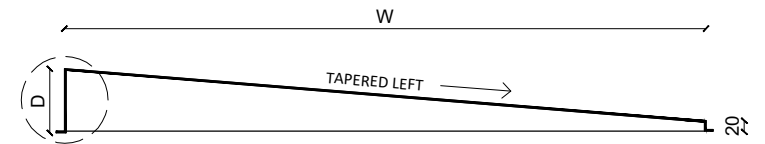
TEGO® MODULE SIZES
