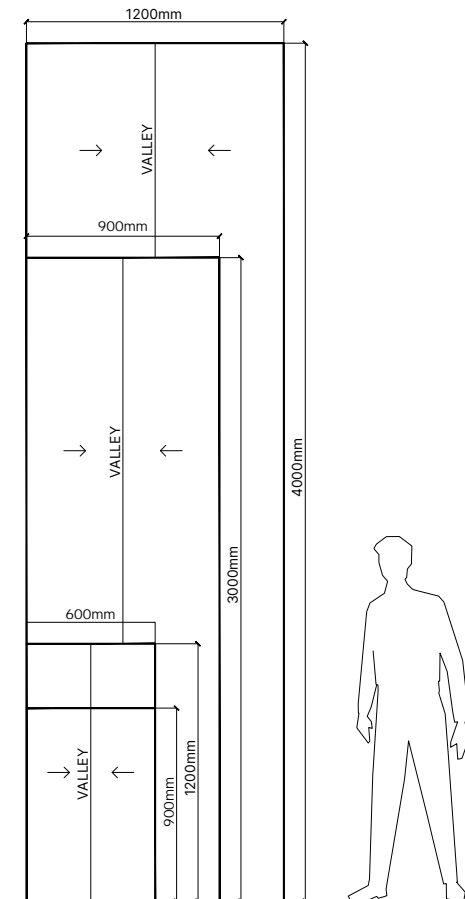
TEGO® MODULE SIZES
