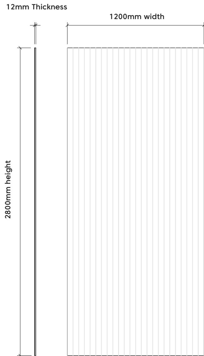
Elevation
