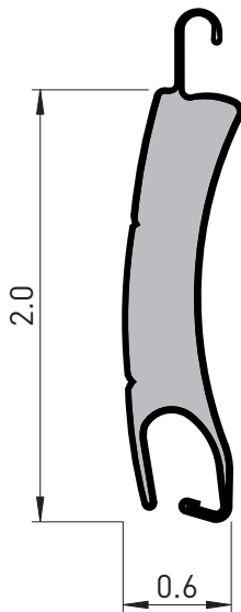
heroal RS 53 RC 2 Scale 1:1
